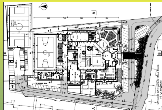
Centro Polivalente - Villanova d'Asti (AT)
